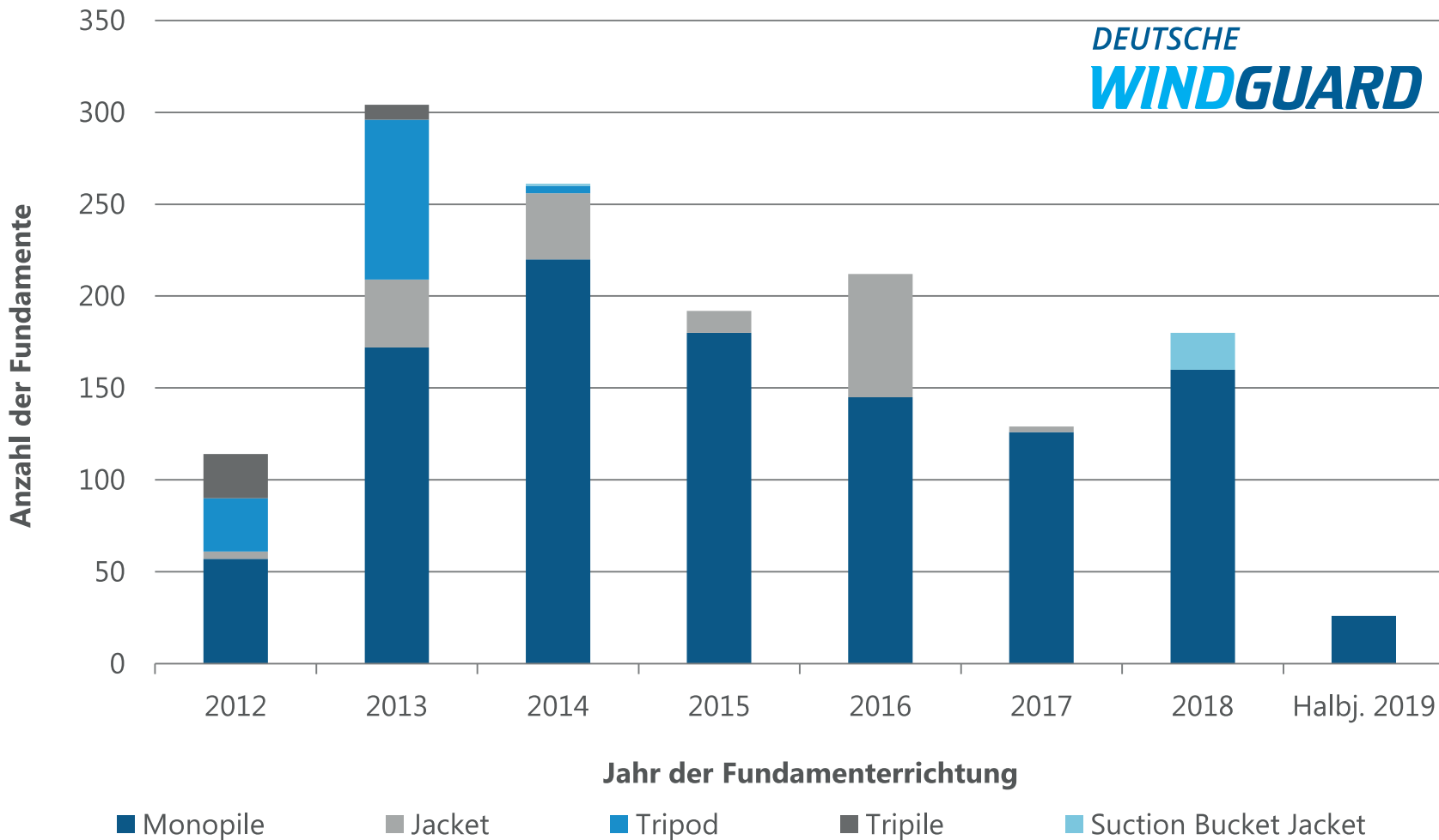
Verwendete Fundamenttypen im Zeitverlauf
